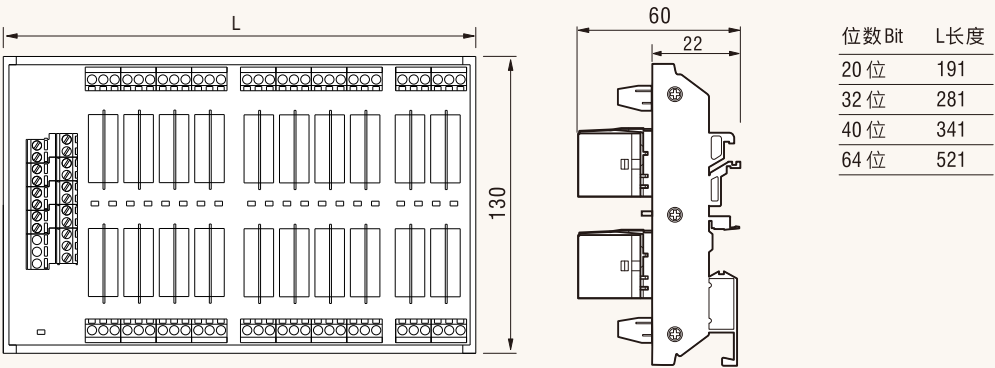
配线图 Wiring Diagram
